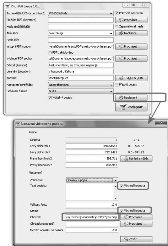
Obrázek 6-52 Příklad nastavení viditelného podpisu
