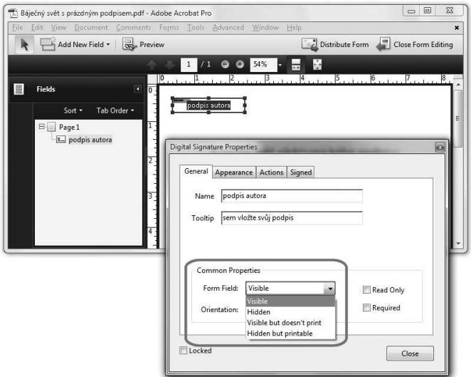
Obrázek 6-81 Volba toho, zda pole i budoucí podpis budou viditelné či nikoli
